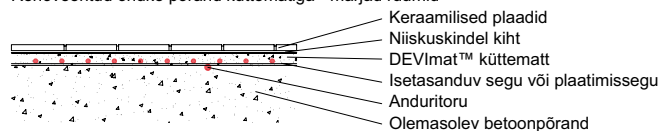
Renoveeritud õhuke põrand küttematiga - märjad ruumid
