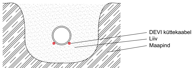
Küttegaabel maa sees paikneval torul
