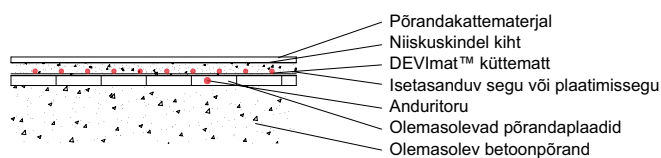
Renoveeritud õhuke põrand küttematiga - kuivad ruumid
